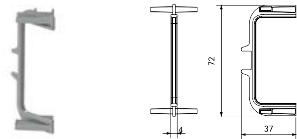
Angolo esterno 90° G13 in plastica Plastic 90° external corner for G13
