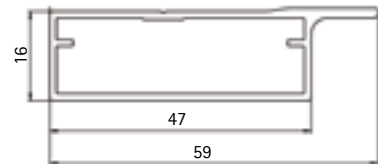
Profilo con maniglia 16x59 Handle profile 16x59
