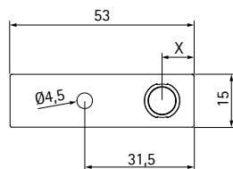
X da 7,5 a 23mm X from 7,5 to 23mm
