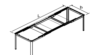
Struttura allungabile a doppia estrazione Extensible structure with double rail adjustment
