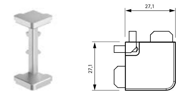
Angolo esterno alluminio 90° G63 90° external aluminum corner G63
