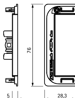
Set tappi terminali esterni in plastica External plastic end cap set
